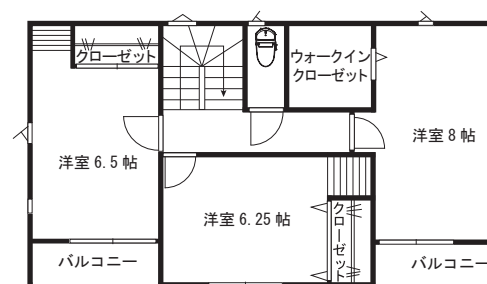
【2階平面図】
