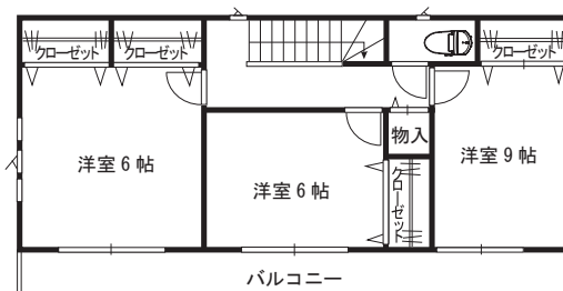
【2階平面図】
