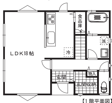
【1階平面図】
