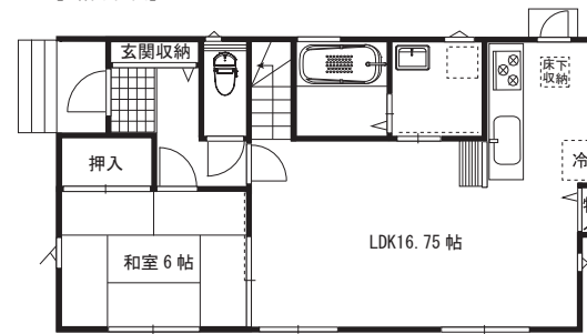
【1階平面図】
