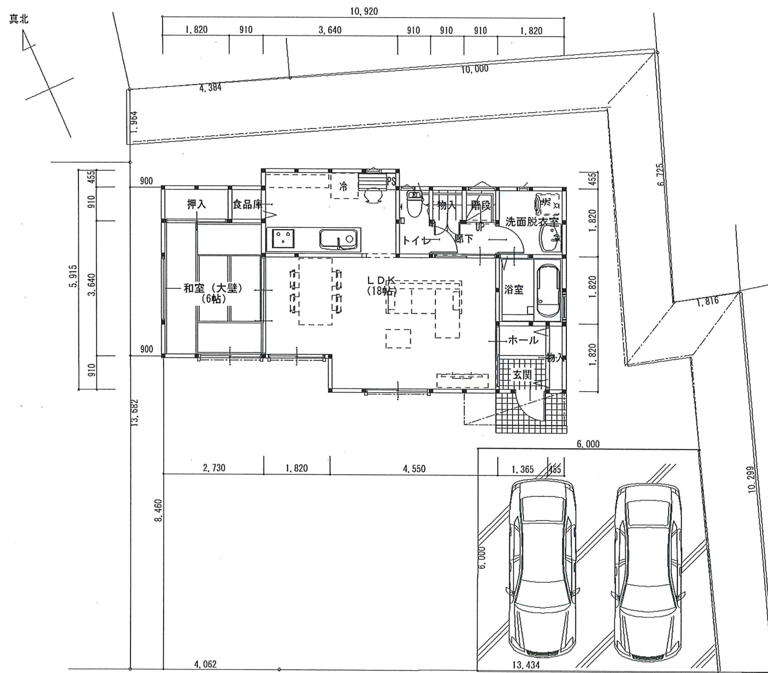
1 階平面図
